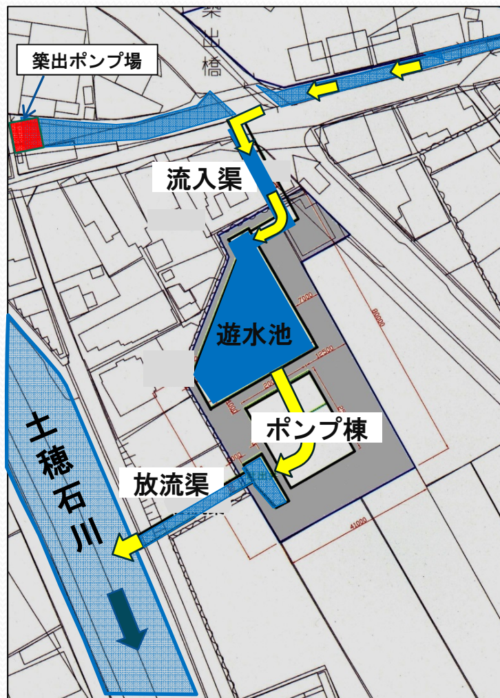
＜参考写真＞ 古開作雨水ポンプ場 & 遊水池
